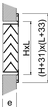
TRV-S
